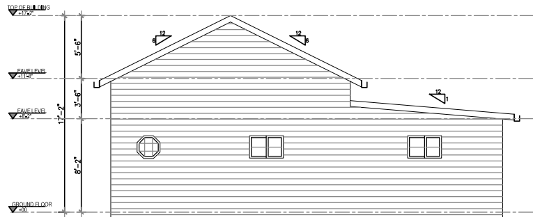
2 REAR ELEVATION Scale: 1"=18"
